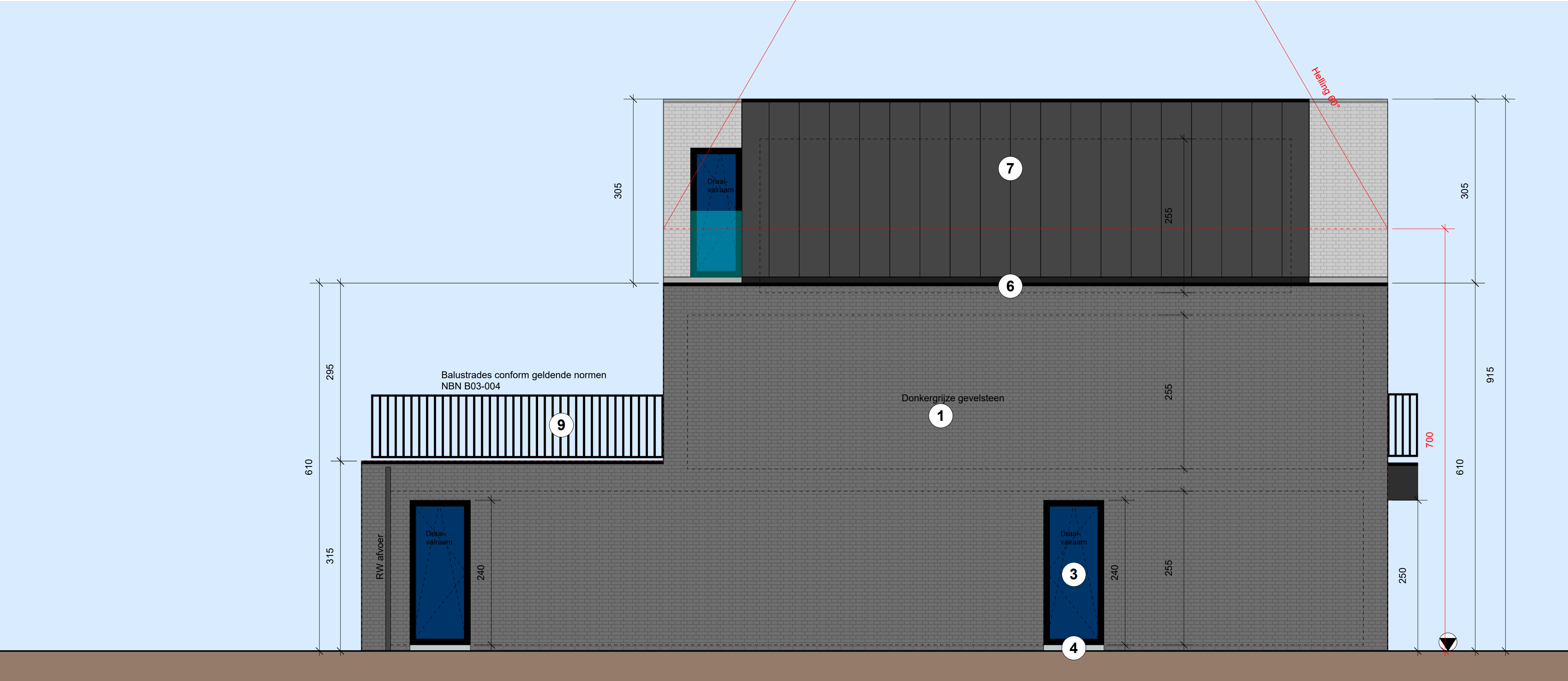
Zijgevelaanzicht links schaal 1/50
