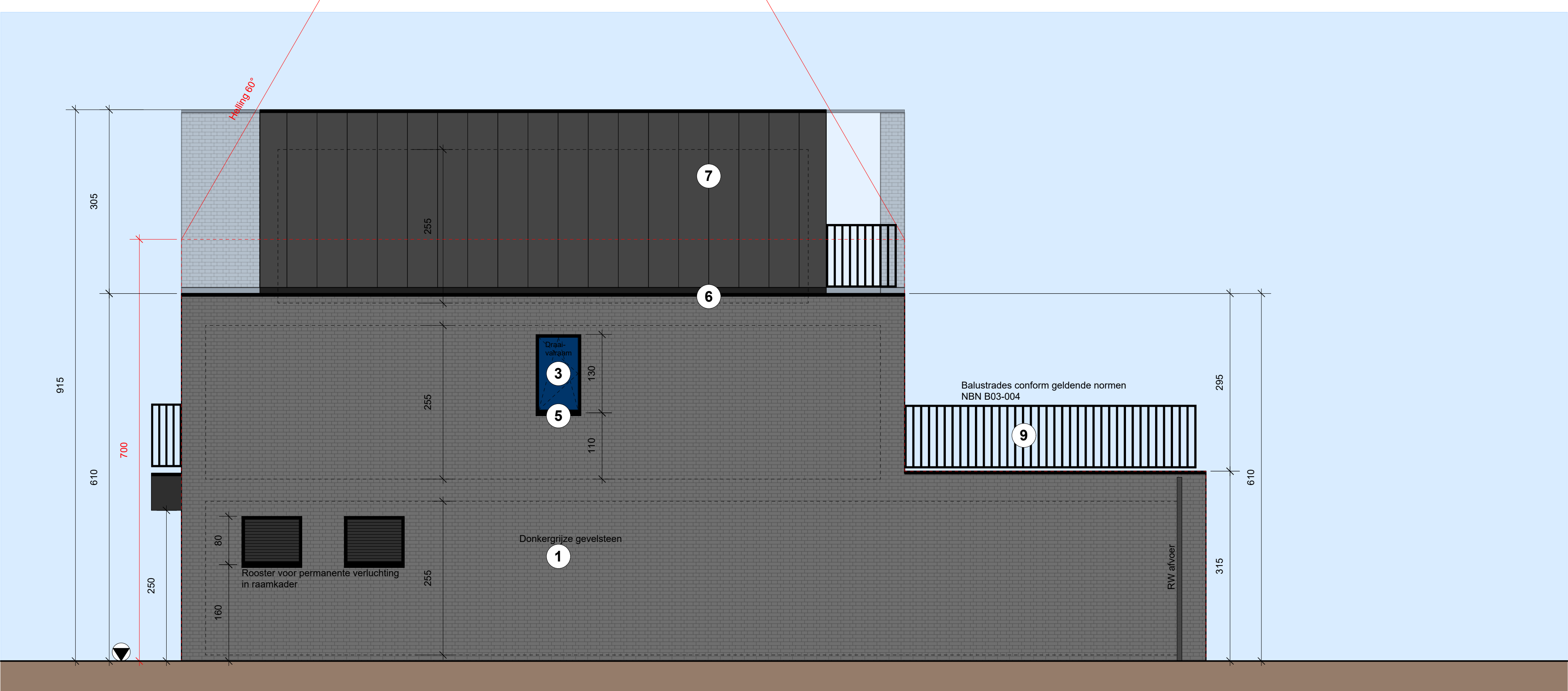
Zijgevelaanzicht rechts schaal 1/50
