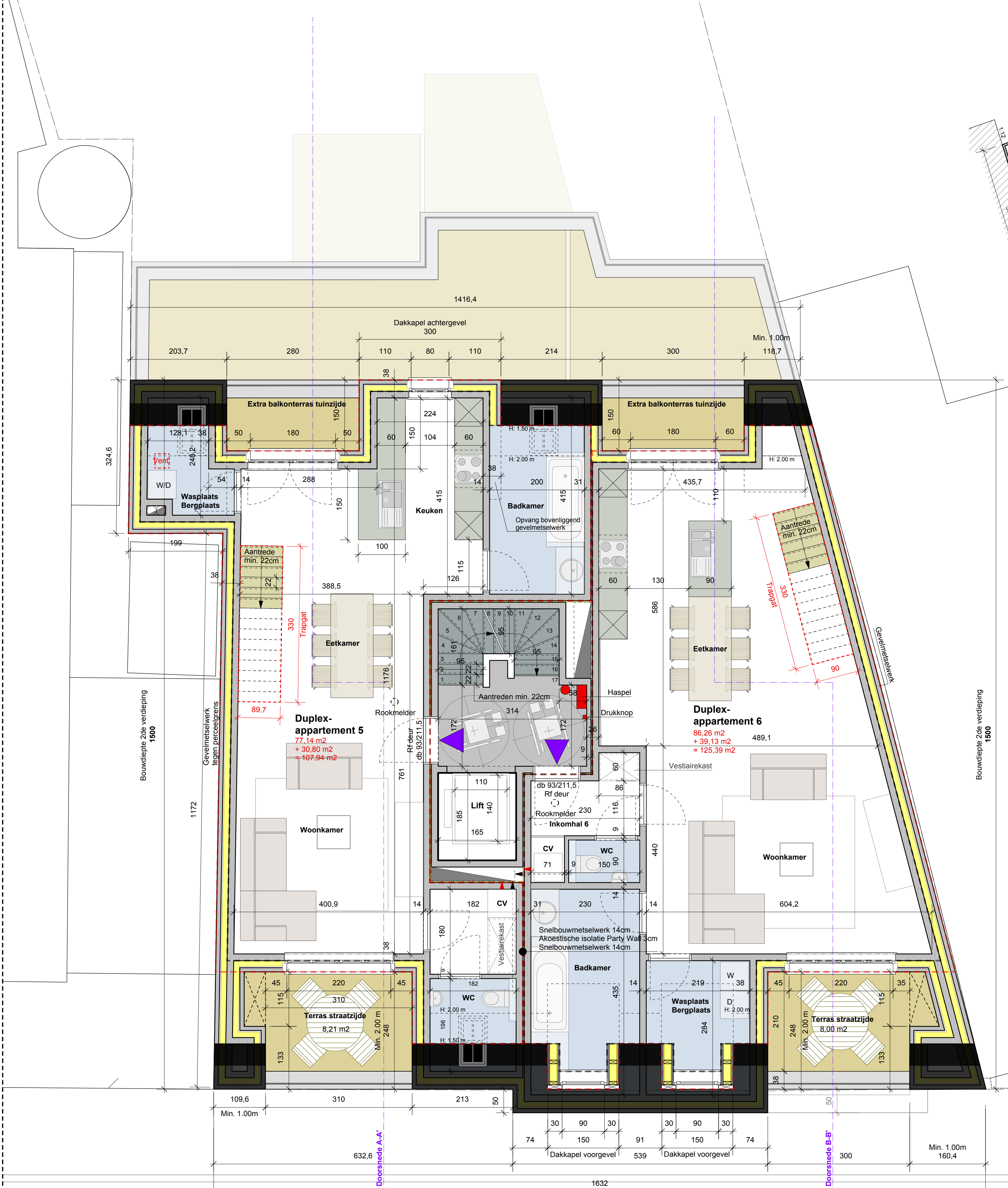
2de verdieppingsplan schaal 1/50
