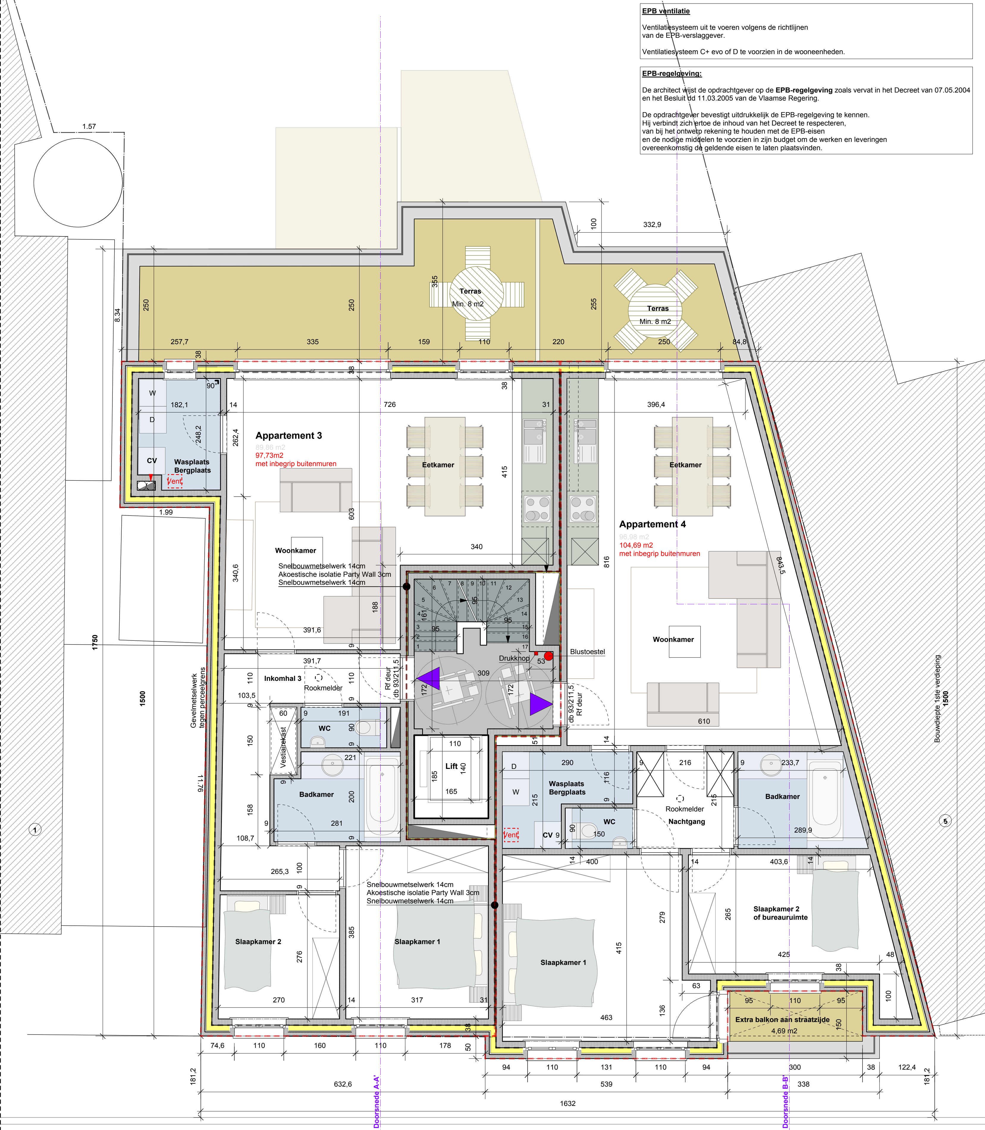
1ste verdieppingsplan schaal 1/50
