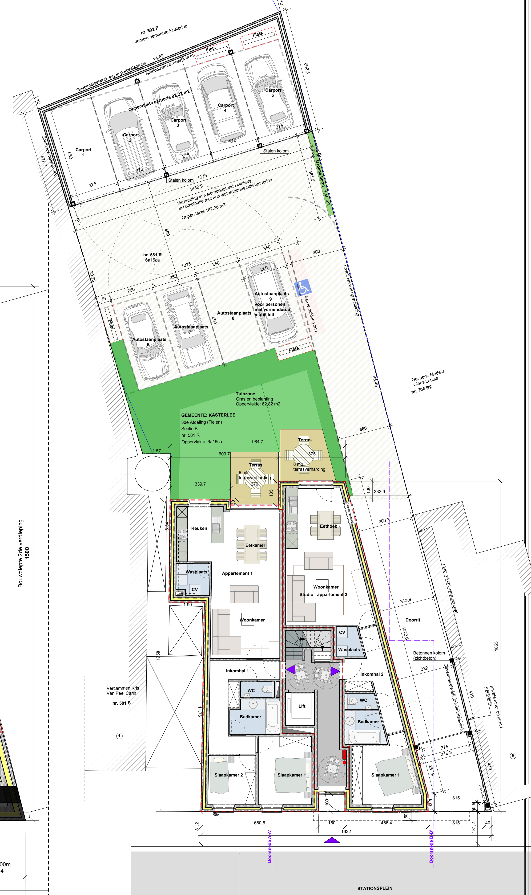
Inplantingsplan na de werken schaal 1/100
