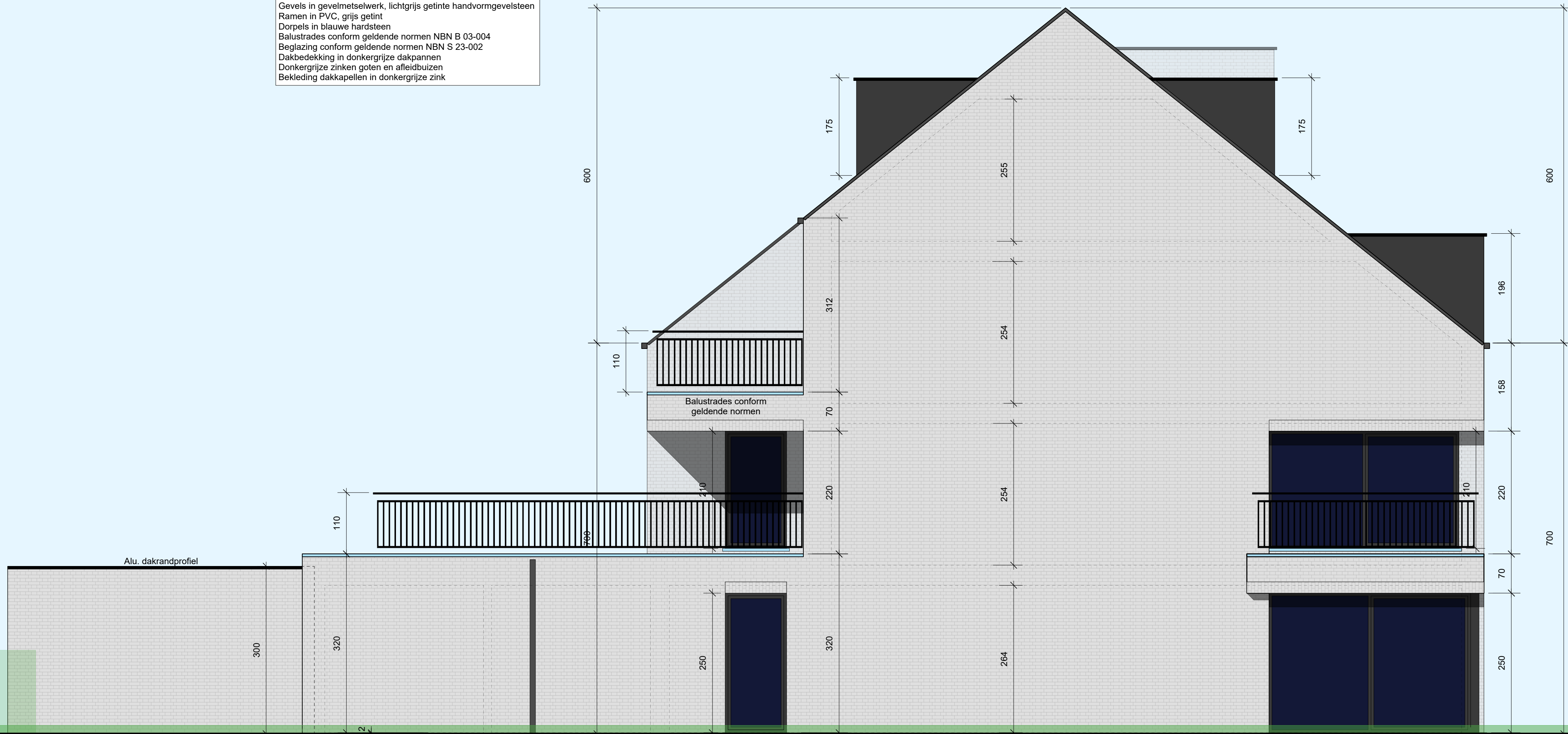
Zijgevelaanzicht links fietsenstalling schaal 1/50
